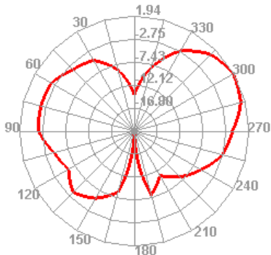
2160.000MHz E1
