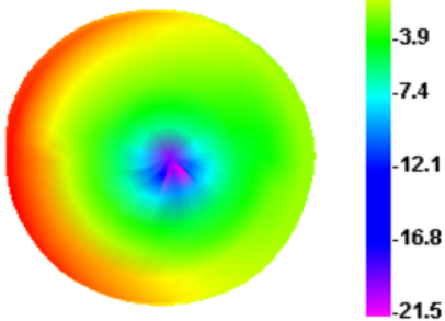
2160.000MHz E1
