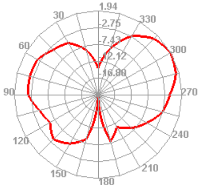
2160.000MHz E1
