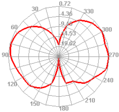
1920.000MHz E1
