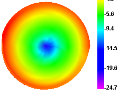
1920.000MHz E1
