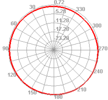
1920.000MHz H
