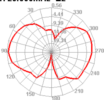
1720.000MHz E2
