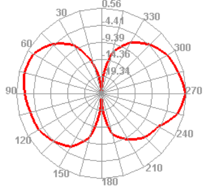
1720.000MHz E1
