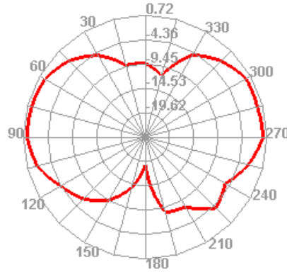
2160.000MHz H
