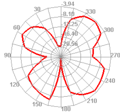
920.000MHz E2
