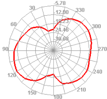
800.000MHz E1
