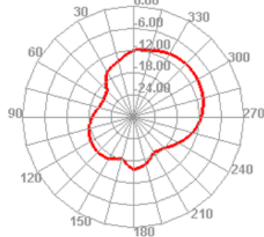
920.000MHz E2
