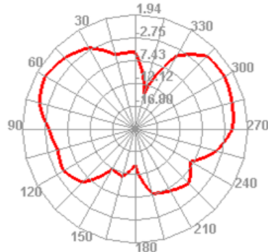
2160.000MHz E2
