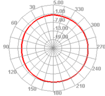
2160.000MHz H
