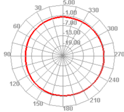
2160.000MHz H
